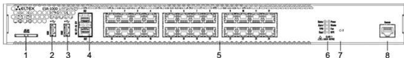
Рисунок 28 – Передняя панель ESR-1000
