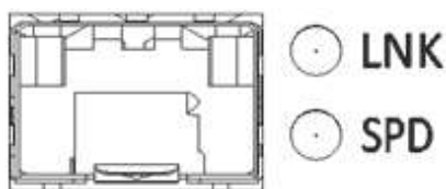
Рисунок 77 – Расположение индикаторов состояния SFP/SFP+-интерфейсов
