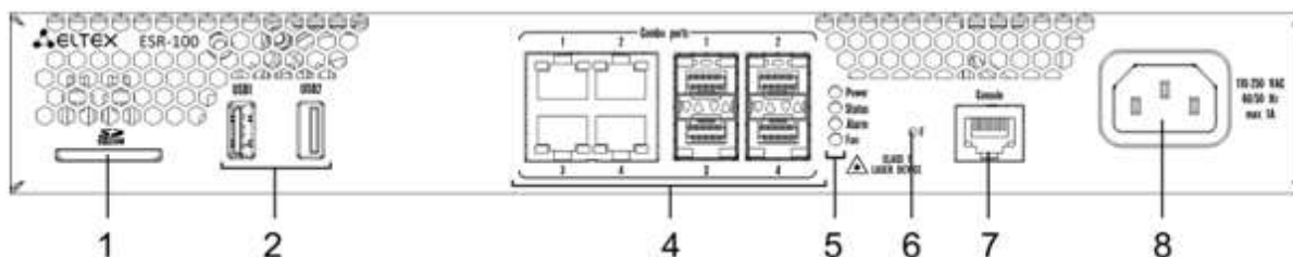
Рисунок 33 – Передняя панель ESR-100
